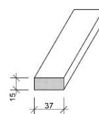
15 x 37 mm REUNALISTA
