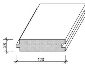
HLL 28 x 120 mm LATTIALAUTA
