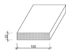
22 x 100 mm KIINNITYSLAUTA
